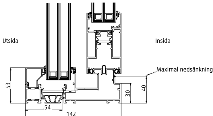
2-spårsprofil för skjutbart system med Köldbryggebrytning.
