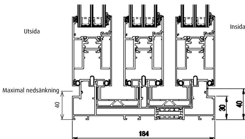
3-spårsprofil för skjutbart system med Köldbryggebrytning.
