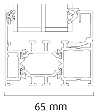
Profil för fast system.
