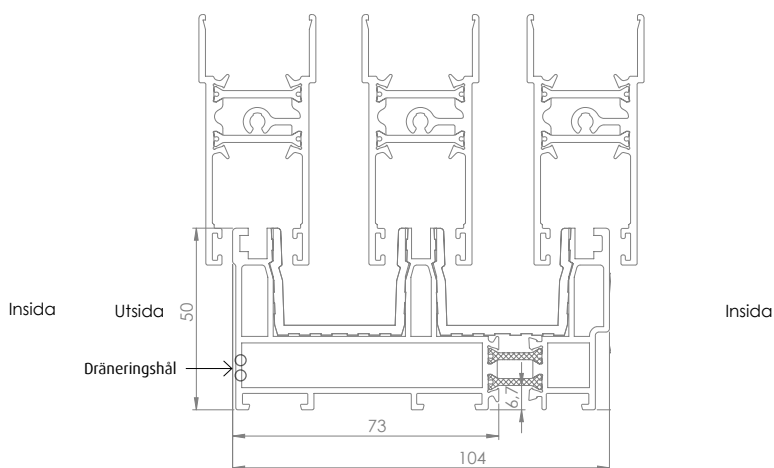
3-spårs profil
