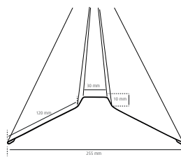
Nockplåt Plåt för sadeltakslösning
